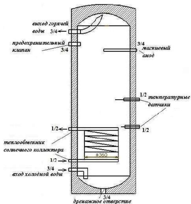
Бак с 1 теплообменником
