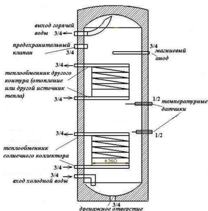
Бак с 2 теплообменниками
