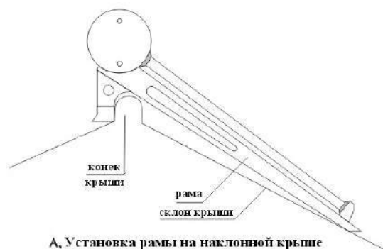
А. Установка рамы на наклонной крыше
